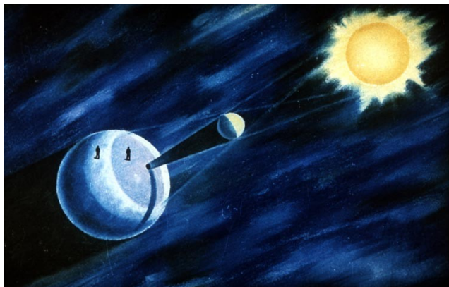
Рис. 1. Схема солнечного затмения
