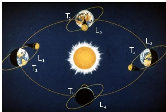
Рис. 2. Условия возможности наступления затмений
